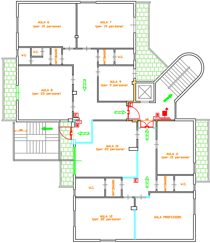
PIANTA PRIMO PIANO EDIFICIO PRINCIPALE
