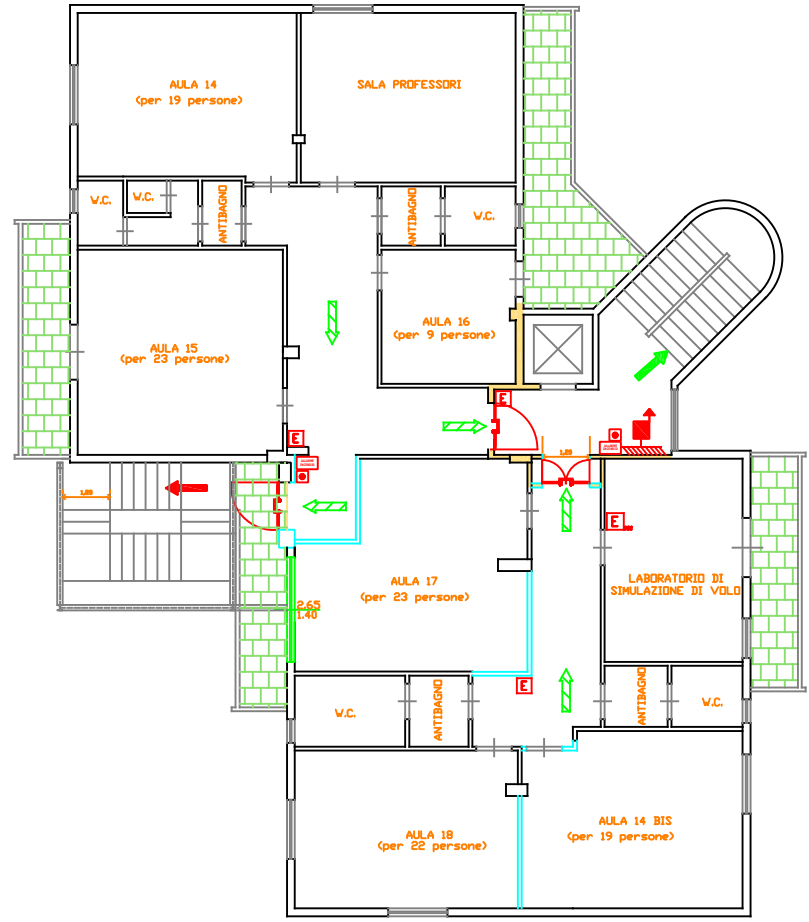
PIANTA SECONDO PIANO EDIFICIO PRINCIPALE
