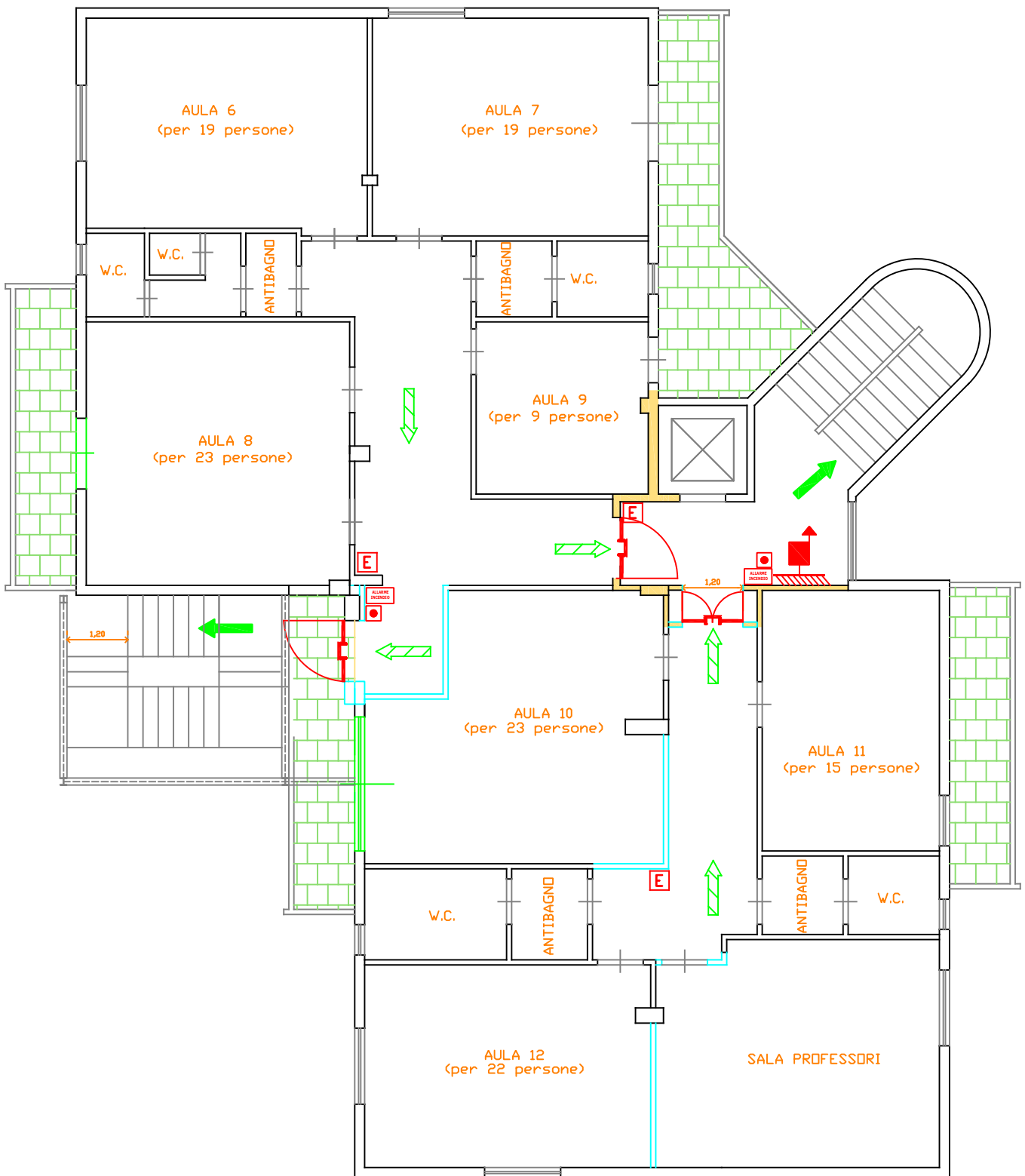
PIANTA PRIMO PIANO EDIFICIO PRINCIPALE
