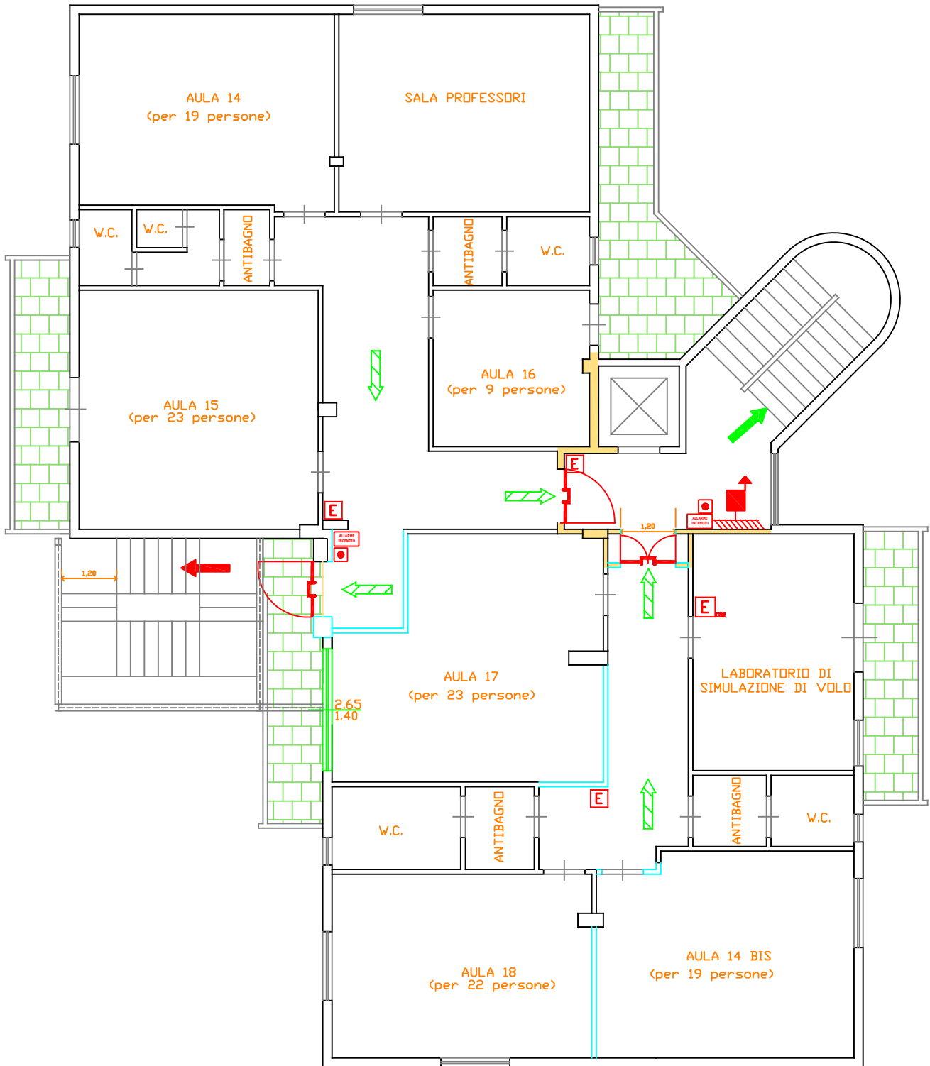
PIANTA SECONDO PIANO EDIFICIO PRINCIPALE
