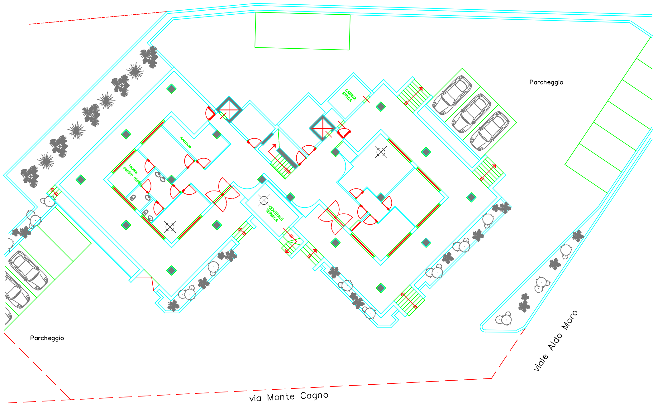
Pianta piano terra e sistemazioni esterne Scala 1:100
